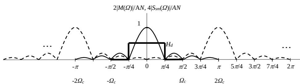
Figure 10 – The spectrum of the signal at the output of the multiplier Рис. 10 – Спектр сигнала на выходе умножителя Слика 10 – Спектар сигнала на излазу множача
