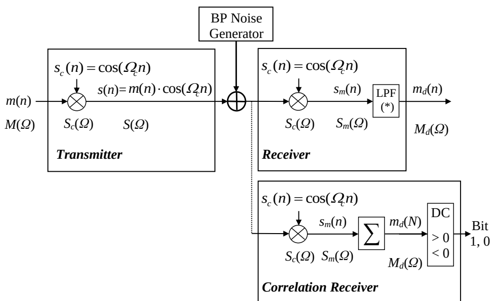
Figure 1 – Discrete communication system Рус. 1 – Дискретная система связи Слика 1 – Дискретни телекомуникациони систем
