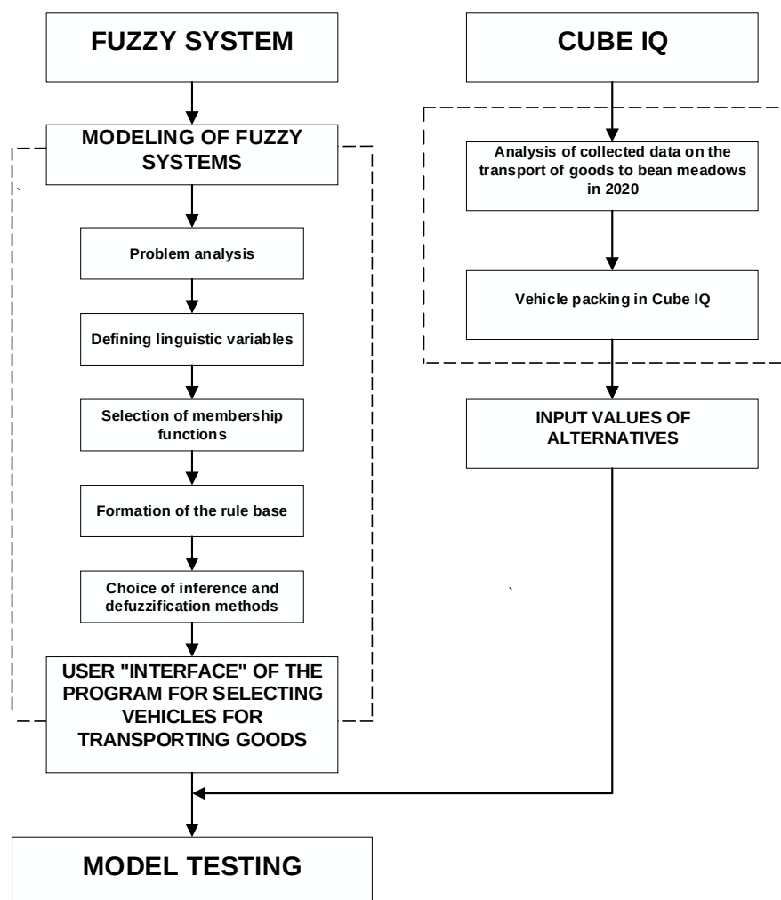
Figure 4 – Scheme of the model for the optimization of vehicle selection Рис. 4 – Схема модели оптимизации выбора транспортных средств Слика 4 – Шема модела за оптимизацију избора возила
