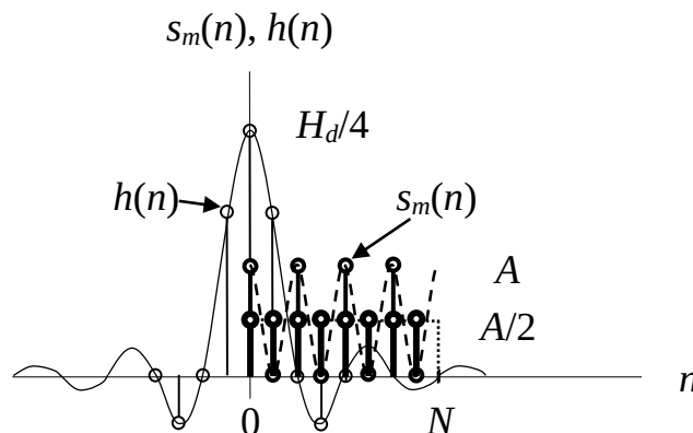
Figure 11 – Convolution of the signals Рис. 11 – Свёртка сигналов Слика 11 – Конволуција сигнала
