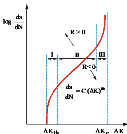
Figure 1 – Typical appearance of the fatigue crack growth curve as a function of \Delta K Рус. 1 – Типичный вид кривой роста усталостной трещины в функции от \Delta K Слика 1 – Типичан изглед криве раста заморне прслине у функцији од \Delta K
