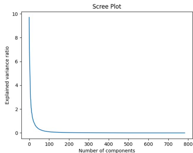
Figure 6a – Scree plot of the explained variance ratio for each component Рис. 6а – График осыпи объясненной дисперсии по каждому компоненту Слика 6а – Scree plot објашњене варијансе за сваку компоненту
