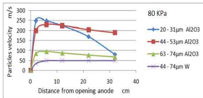
Figure 1 – Average velocities of \text{Al}_2\text{O}_3 and W particles at a pressure of 80kPa Рис. 1 – Средняя скорость частиц \text{Al}_2\text{O}_3 и W под давлением 80KPa Слика 1 – Средње брзине честица \text{Al}_2\text{O}_3 и W при притиску од 80 KPa
