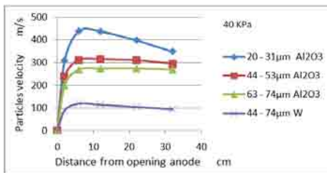
Figure 2 – Average velocities of \text{Al}_2\text{O}_3 and W particles at a pressure of 40KPa Рис. 2 – Средняя скорость частиц \text{Al}_2\text{O}_3 и W под давлением 40KPa Слика 2 – Средње брзине честица \text{Al}_2\text{O}_3 и W при притиску од 40 KPa
