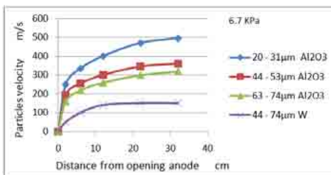
Figure 3 – Average velocities of \text{Al}_2\text{O}_3 and W particles at a pressure of 6.7 KPa Рис. 3 – Средняя скорость частиц \text{Al}_2\text{O}_3 и W под давлением 6,7 Кра Слика 3 – Средње брзине честица \text{Al}_2\text{O}_3 и W при притиску од 6,7 KPa
