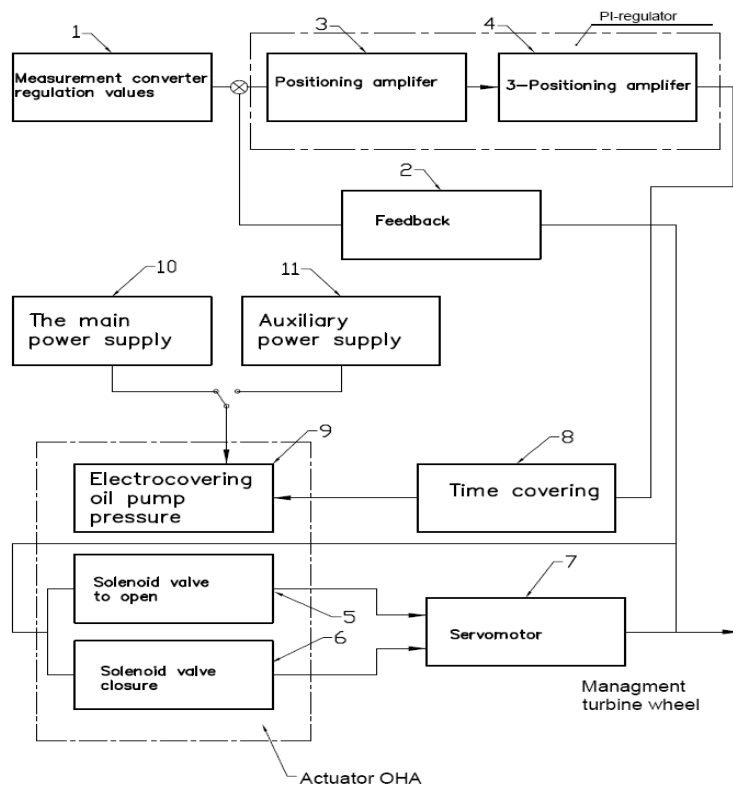
Figure 6 – Electro hydraulic controller type EHR-80 for MHPs Рисунок 6 – Электрогидравлический регулятор ЭГР-80 для Мини ГЭС Слика 6 – Електрохидраулични регулатор тип EHR-80 за МНЕ
