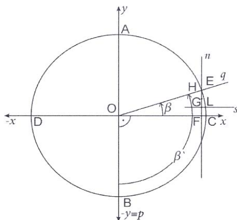
Figure 13 – Potation of \beta' for the angle (-90^\circ) Рис. 13 – Поворот угла \beta' на (-90^\circ) Слика 13 – Ротација угла \beta' за (-90^\circ)
