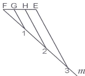
Figure 11 – Division of the length FE for the angle trisection of \beta < 22^\circ 30' Рис. 11 – Деление отрезка FE по трисекции угла \beta < 22^\circ 30' Слика 11 – Подјела дужи FE за трисекцију угла \beta < 22^\circ 30'
