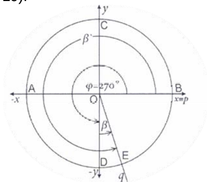
Figure 18 – Arm q of the \beta' angle belongs to the fourth quadrant Рис. 18 – Луч q угла \beta' принадлежит четвертому квадранту Слика 18 – Крак q угла \beta' припада четвртном квадранту
