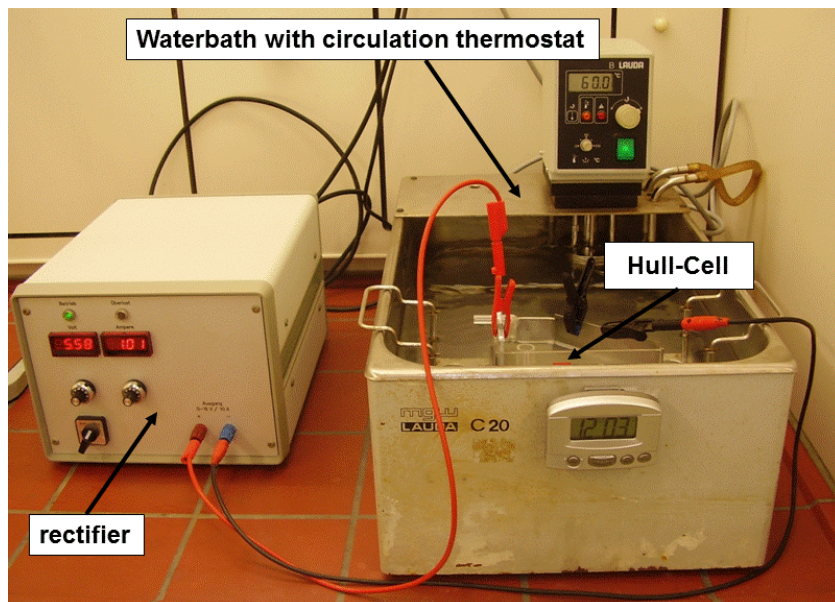
Figure 2 – Electroplating in the Hull cell Рус. 2 – Гальванизация в ячейке Хулл Slika 2 – Galvanizacija u Hulovoj ćeliji
