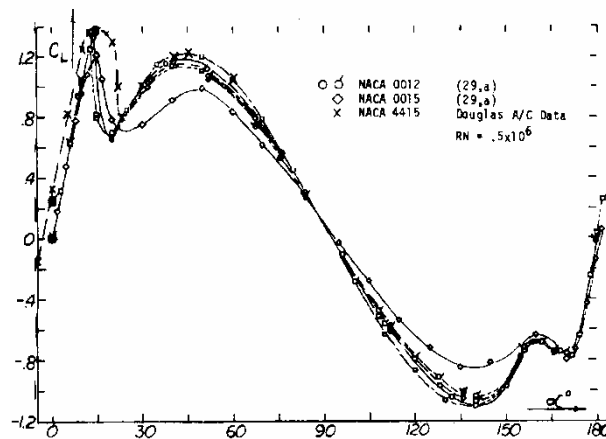
Figure 21 – Variations of the lift coefficient for \alpha = 0^\circ - 180^\circ Рус. 21 – Вариации значений коэффициента подъемной силы при \alpha = 0^\circ - 180^\circ Slika 21 – Varijacije koeficijenta uzgona za \alpha = 0^\circ - 180^\circ
