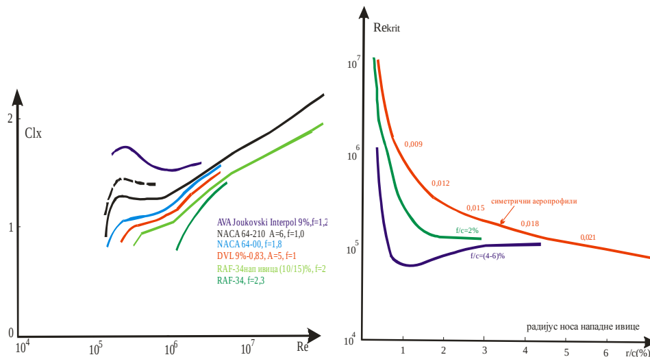
Figure 15 – Maximum lift of rectangular wings as a function of Re , t/c = 8-10\% Рус. 15 – Максимальная подъемная сила прямоугольного крыла как функция Re , t/c = 8-10\% Slika 15 – Maksimalni uzgon pravougaonih krila kao funkcija Re , t/c = 8-10\%
