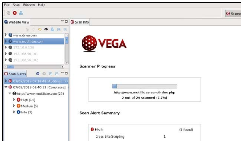
Figure 16 – Vega – scanning Рис. 16 – Vega – сканирование Slika 16 – Vega – skeniranje
