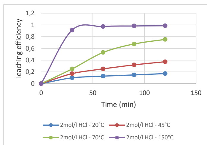
Figure 4 – Influence of temperature and time on the yttrium dissolution Рус. 4 – Влияние температуры и времени на процесс растворение иттрия Slika 4 –Uticaj temperature i vremena na rastvaranje itrijuma
