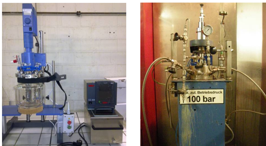
Figure 3 – a) a glass reactor b) an autoclave Рис. 3 – а) стеклянный реактор б) автоклав Slika 3 – a) stakleni reaktor b) autoklav
