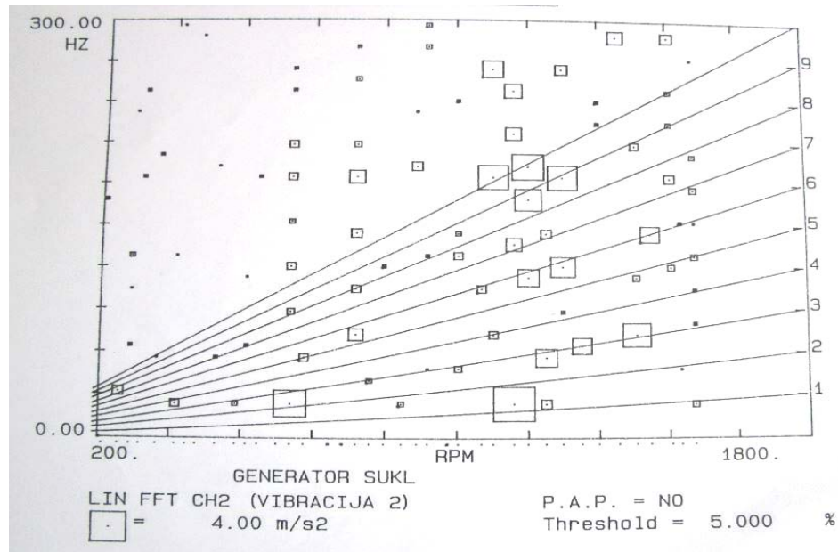
Figure 9 – Campbell diagram, FFT, Syy, bearing L2 Рус. 9 – Диаграмма Кэмпбелла, FFT, Суу, подшипник L2 Slika 9 – Campbell-ov dijagram, FFT, Syy, ležaj L2
