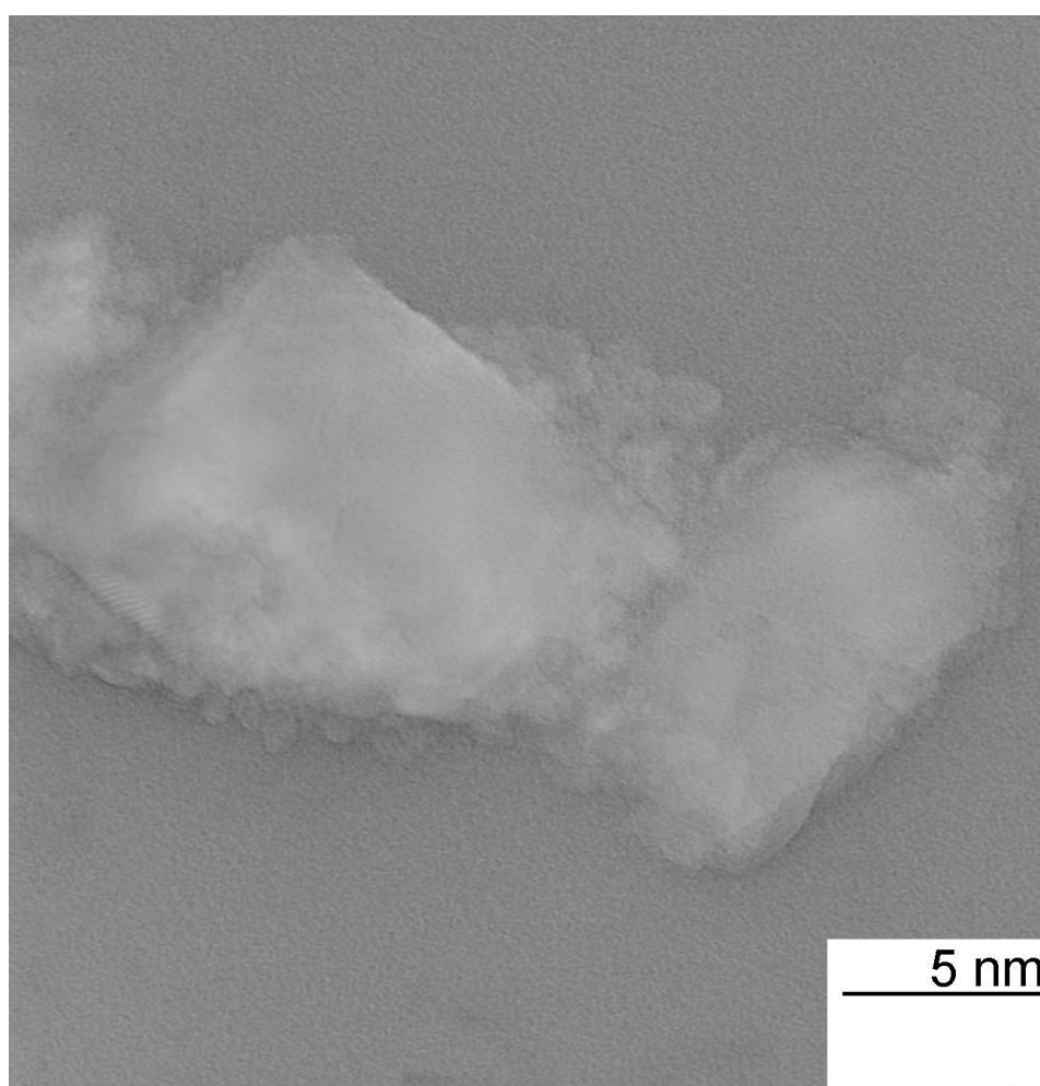
Slika 2 – Fotografija dobijena pomoću TEM-a za uzorak S_1 nanočestičnog \gamma\text{-Fe}_2\text{O}_3 Figure 2 – Transmission electron micrograph for the S_1 sample of the nanoparticle \gamma\text{-Fe}_2\text{O}_3
