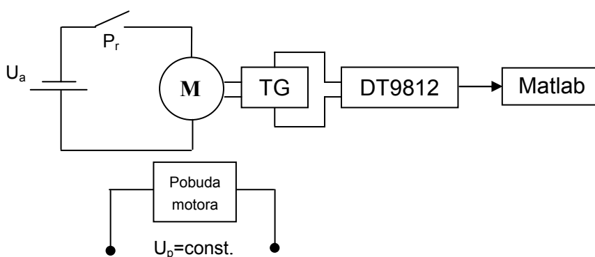
Slika 5 – Principalska šema za identifikaciju jednosmernog motora
