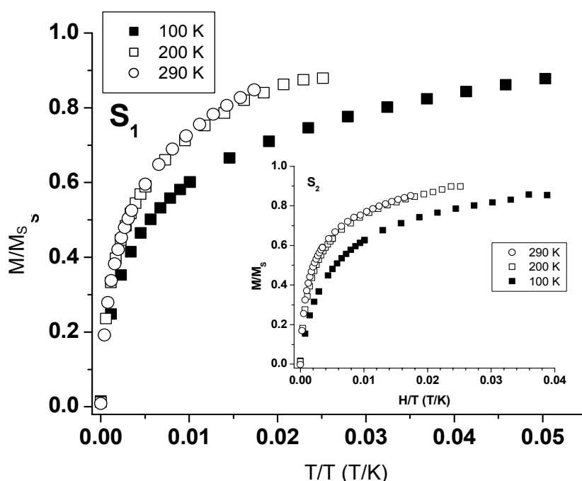
Slika 9 – Zavisnost M/M_s od H/T za uzorke nanočestičnog maghemita
