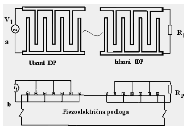
Slika 2 – Šematski prikaz transversalnog PAT filtra tipa linije za kašnjenje
