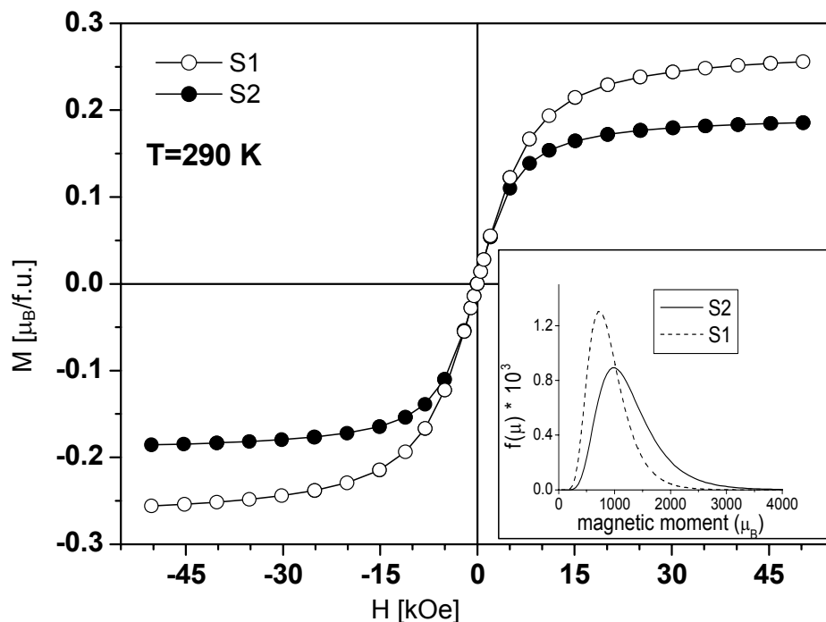
Slika 7 – Zavisnost magnetizacije od magnetnog polja na temperaturi 290 K. Punom linijom su prikazane modificovane Langevin-ove krive dobijene podešavanjem izraza (5) na eksperimentalne vrednosti za uzorke S 1 i S 2
