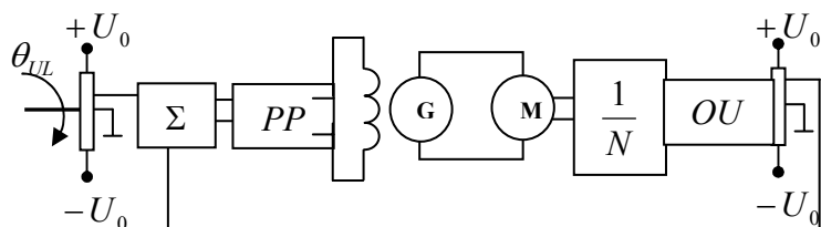
Slika 1 – Principna šema potencijometarskog pozicionog servosistema
