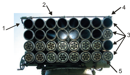
Slika 2 – Mehanizam AKR-a:
