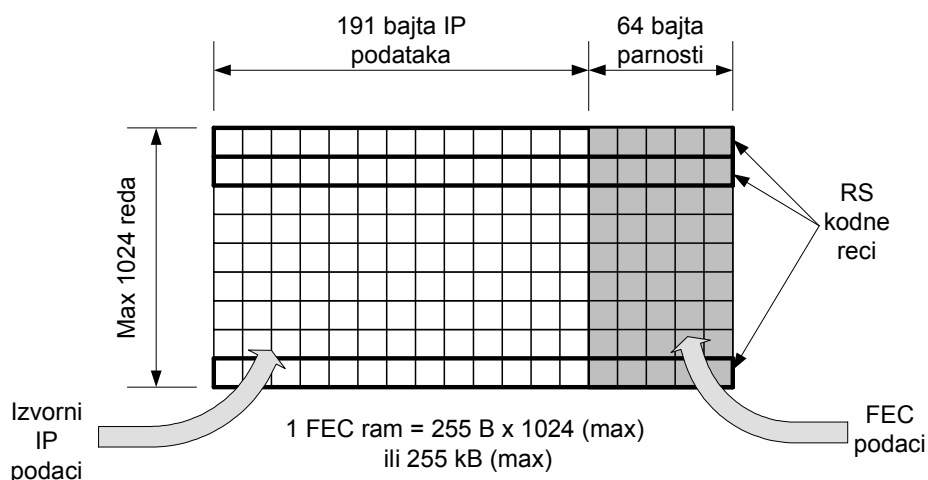
Slika 7 – Struktura MPE-FEC rama
