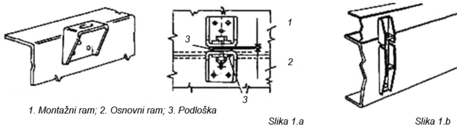
Slika 1 – Primer konzolne veze osnovnog i montažnog rama
