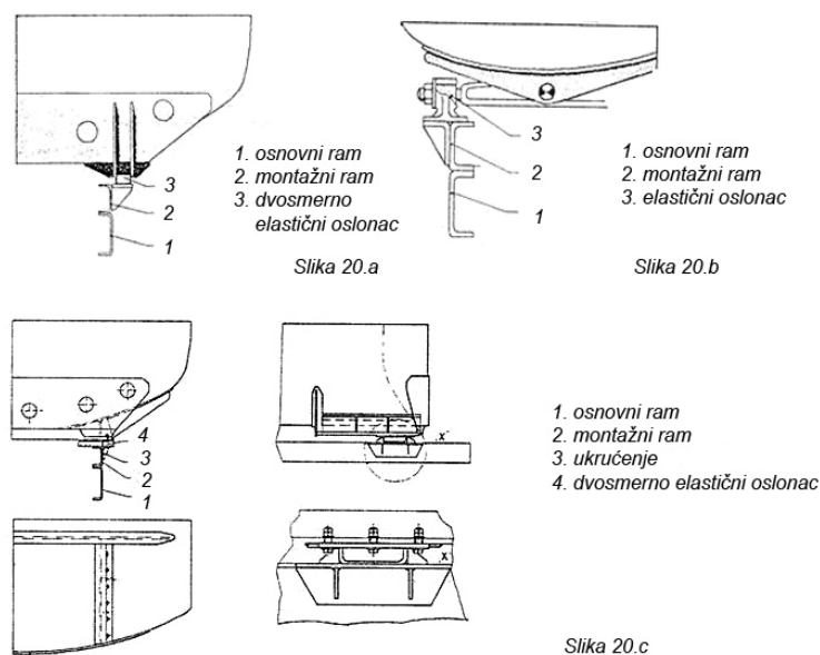
Slika 20 – Instrukcija za nadgradnju proizvođača „Mercedes – Benz“
