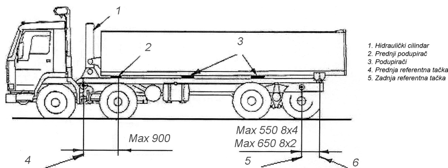
Slika 13 – Četveroosovinski kiper proizvođača „Volvo“ koji istovaruje unazad
