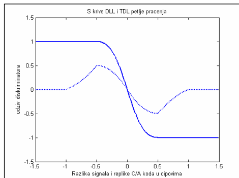
Slika 11 – Odziv diskriminatora DLL i TDL petlje praćenja
