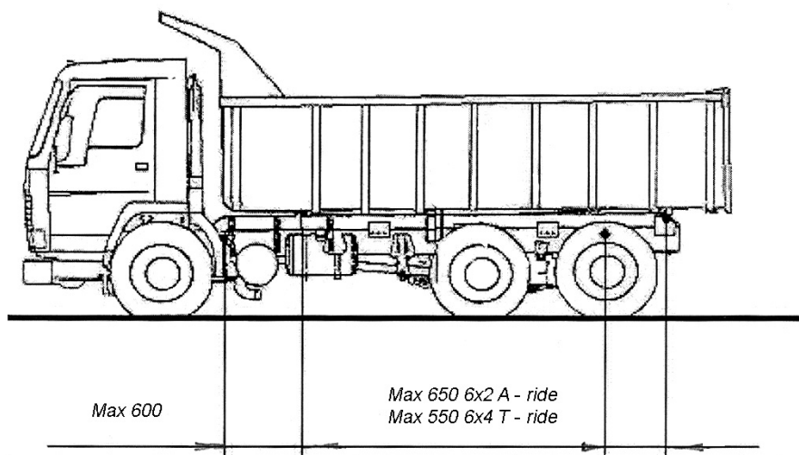
Slika 12 – Troosovinski kiper proizvođača „Volvo“ koji istovar vrši unazad
