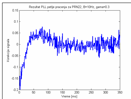
Slika 17 – Signal na izlazu PLL za PRN22, B=10\text{ Hz} , \gamma=0.3
