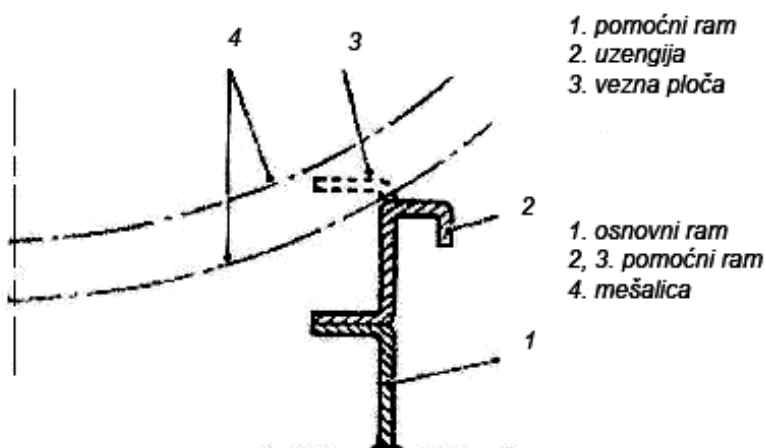
Slika 8 – Instrukcije proizvođača „Mercedes“ za nadgradnju automešalice
