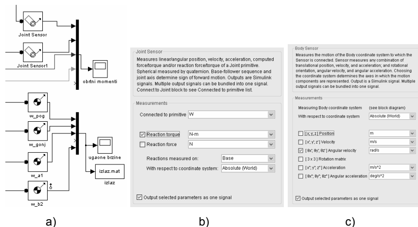
Slika 14 – a) Podsystem za praćenje rezultata simulacije; b) i c) Definisanje rada davača obrtnog momenta i ugaone brzine
