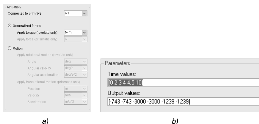
Slika 5 – a) Parametri za izbor veličine za pobuđivanje u Joint Actuator-u; b) Parametri za definisanje obrtnog momenta motora Figure 5 – a) Parameters for the selection of the size of the excitation in the Joint Actuator; b) Parameters to define the engine torque
