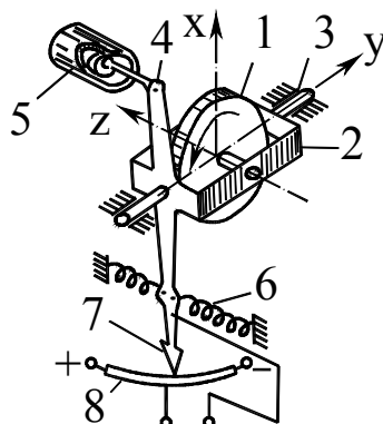
Slika 22 – Brzinski žiroskop
