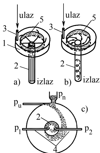
Slika 24 – Šema i princip rada pneumoničnog brzinskog žiroskopa
