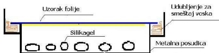
Slika 3 – Šematski prikaz metalne posudice sa uzorkom folije
