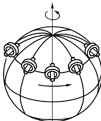
Slika 20 – Ponašanje žiroskopa podešenog prema Zemlji
