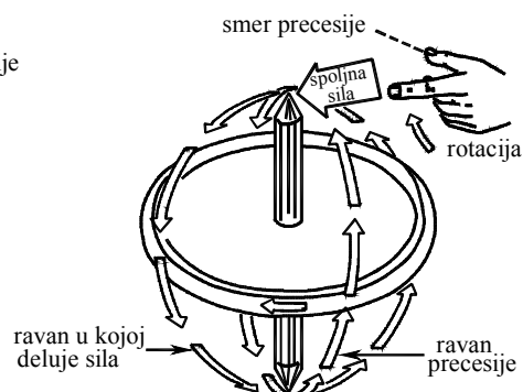
Slika 15 – Precesija žiroskopa
