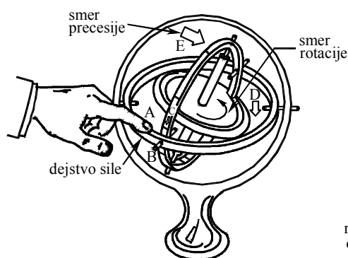
Slika 14 – Određivanje pravca precesije žiroskopa
