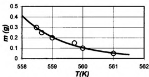
Slika 5 – Uticaj mase uzorka na temperaturu paljenja TNT-a
