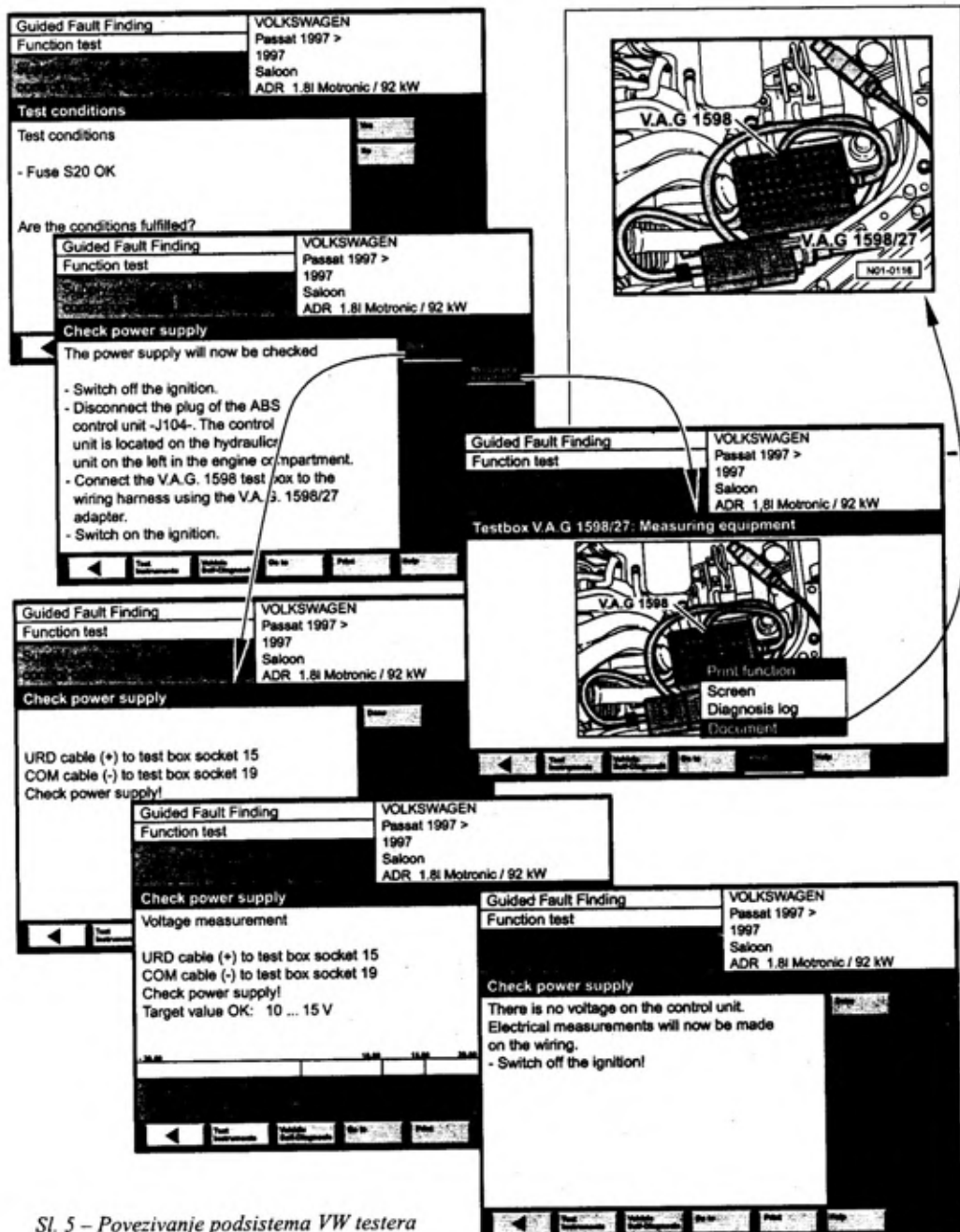
Sl. 5 – Povezivanje podsistema VW testera
