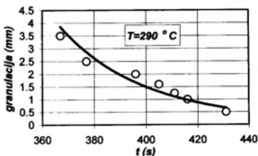
Slika 6 – Rezultati merenja uticaja granulacije uzorka TNT na vreme zadržke
