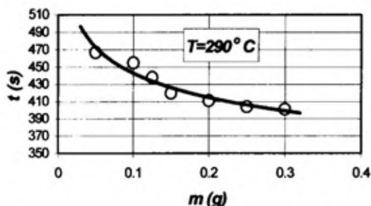
Slika 4 – Uticaj mase uzorka na vreme zadržke za TNT
