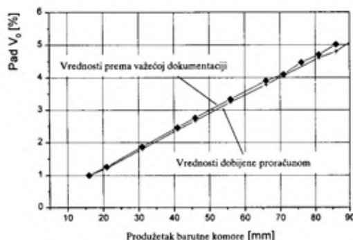
Sl. 4 – Pad početne brzine projektila u zavisnosti od produžetka barutne komore za haubicu 122 mm D30J
