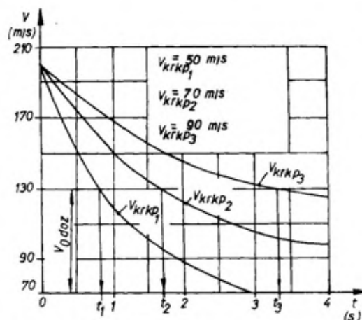
Sl. 8 – Promena vremena kočenja sistema teret-padobran do brzine V_{0doz} u funkciji površine kočćeg padobrana V_{krkp}
