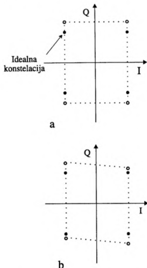
Sl. 4 – Nebalansiranost analognog IQ demodulatora:
