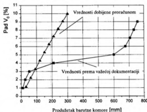
Sl. 5 – Pad početne brzine projektila u zavisnosti od produžetka barutne komore za top 130 mm M46
