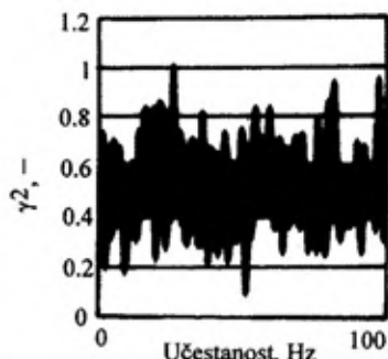
Sl. 9 – Funkcija koherencije: točak upravljača – desni točak, za brzinu vozila 10 m/s (varijanta sa mehaničkim upravljačem)
