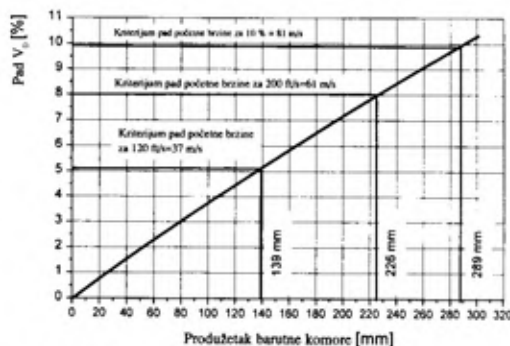
Sl. 6 – Pad početne brzine projektila u zavisnosti od produžetka barutne komore za top-haubicu 152 mm M84
