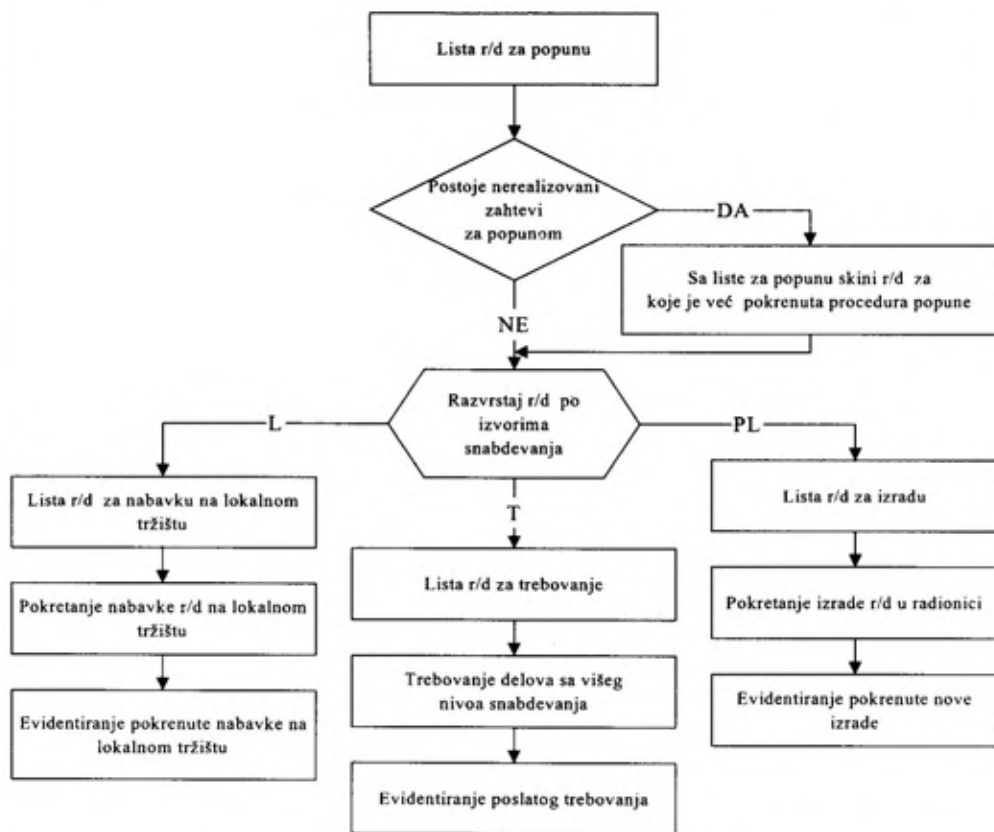
Sl. 6 – Algoritam aktivnosti popune delovima sa liste r/d za popunu
