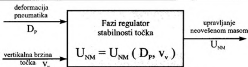
Sl. 14 – Blok-šema fazi regulatora stabilnosti točka
