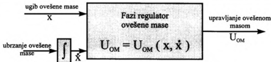
Sl. 12 – Blok-šema fazi regulatora oвеšene mase
