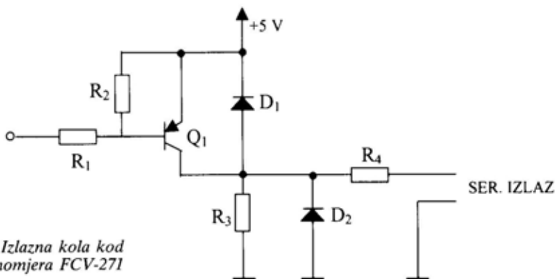
Sl. 3 – Izlazna kola kod žiromkompasa Standard 20
