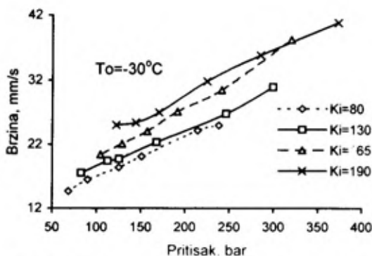
Sl. 11 – Zavisnosti brzine sagorevanja od pritiska za razne odnose A_s/A_p pri temperaturi T_0 = -30^\circ\text{C}
