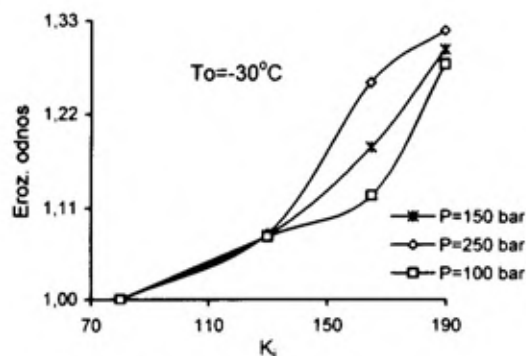
Sl. 17 – Zavisnosti erozivnog odnosa od K_i = A_s/A_p za razne pritiske na T_o = -30^\circ\text{C}
