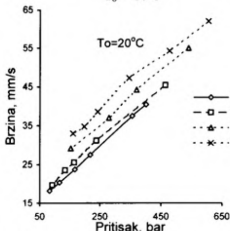
Sl. 9 – Zavisnosti brzine sagorevanja od pritiska za razne odnose A_s/A_p pri temperaturi T_0 = 20^\circ\text{C}
