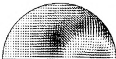
Sl. 5 – Strujno polje u x-y ravni, z = 9 \text{ cm} , na 15^\circ\text{KV} posle SMT
