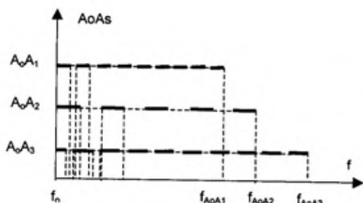
Sl. 5 – Grafički prikaz zavisnosti ugla od noseće frekvencije tri različita radio-signal sa frekvencijskim skakanjem:
