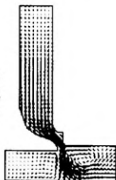
Sl. 4 – Strujno polje u y-z ravni, x = 2 \text{ cm} , na 15^\circ\text{KV} posle SMT (zona usisnog ventila)
