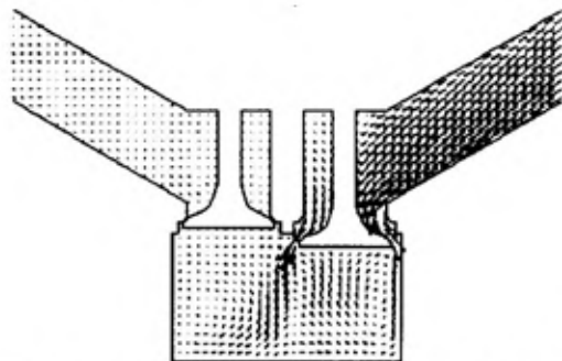
Sl. 6 – Strujno polje u x - z ravni, y = 0 , na 75°KV posle SMT
