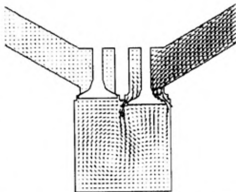
Sl. 8 – Strujno polje u x - z ravni, y = 0 , na 120°KV posle SMT
