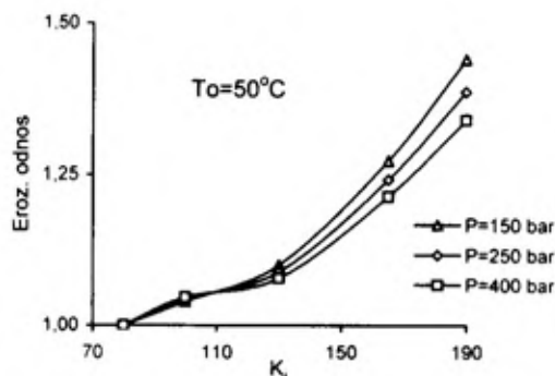
Sl. 18 – Zavisnosti erozivnog odnosa od K_i = A_s/A_p za razne pritiske na T_o = 50^\circ\text{C}
