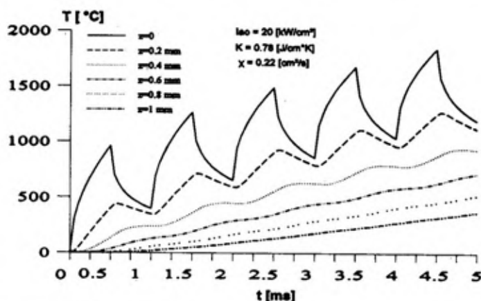
Sl. 10 – Promena temperature u uzorku od gvožđa ozračenim intenzitetom zračenja u obliku niza pravougaonih impulsa
