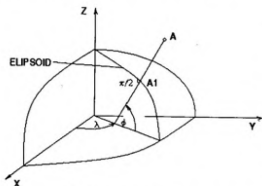
Sl. 2 – Geodetske koordinate tačke A: geodetska longitudina ( \lambda ), geodetska latituda ( \phi ) i geodetska visina (dužina A-A1) tačke A
