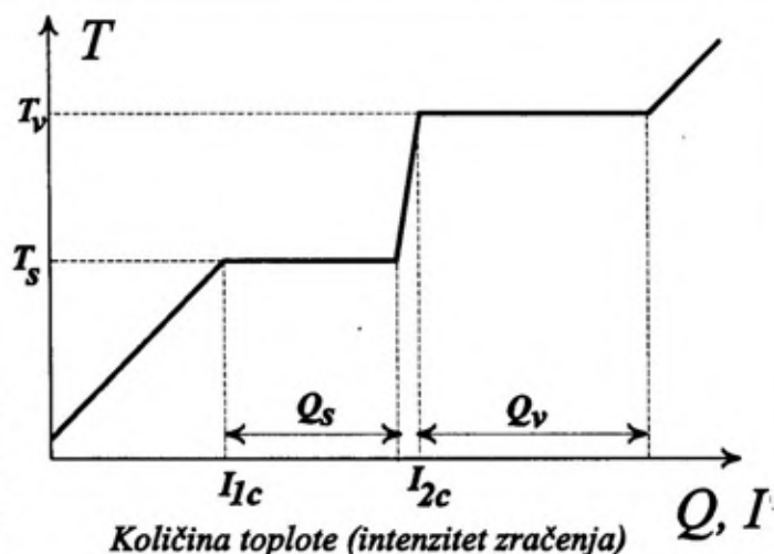
Sl. 14 – Kvalitativni dijagram faznih promena u materijalu:
