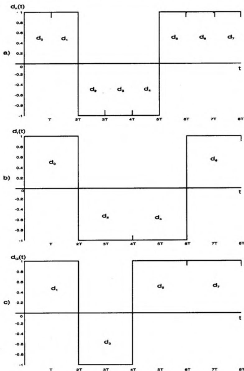
Sl. 1 – Ilustracija kvadraturnih nizova: a) – informacioni niz, b) – niz u fazi, c) – niz u kvadraturi
