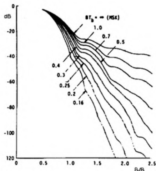
Sl. 9 – Odnos snage signala prelivene u susedne kanale i ukupne snage u posmatranom kanalu
