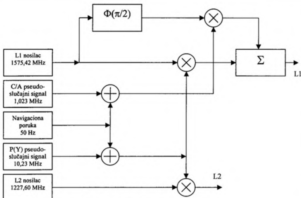
Sl. 3 – Blok-šema formiranja L1 i L2 signala
