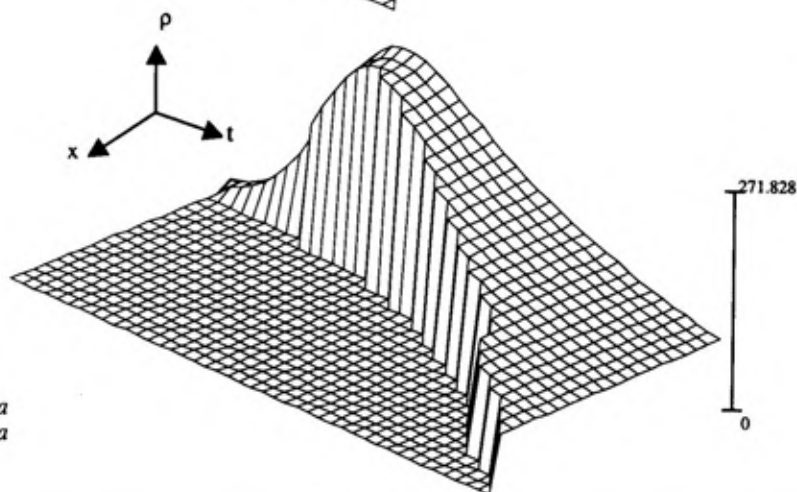
Sl. 3 – Gustina barutnih gasova
