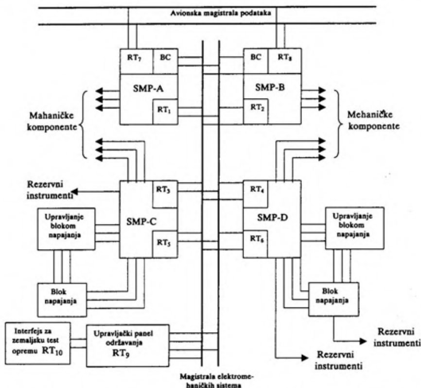
Sl. 6 – Arhitektura sistema integrisanog upravljanja za eksperimentalni avionski program (EAP)
