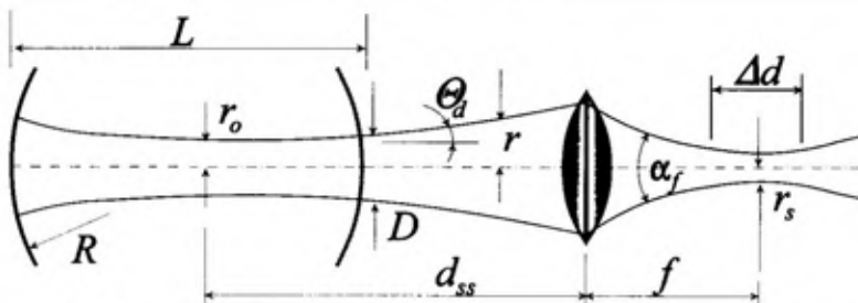
Sl. 2 – Fokusiranje laserskog snopa dobijenog u konfokalnom rezonatoru: L – dužina rezonatora, R – radijus zakrivljenosti ogledala, r – radijus snopa, r_o – radijus struka snopa u rezonatoru, r_s – radijus spota (struka snopa u fokusu), f – fokusna dužina sočiva, D – prečnik izlaznog otvora lasera, \Delta d – dubina fokusiranja, \Theta_d – ugao divergencije, d_{ss} – udaljenost sočiva od struka u rezonatoru, \alpha_f – ugao fokusiranja
