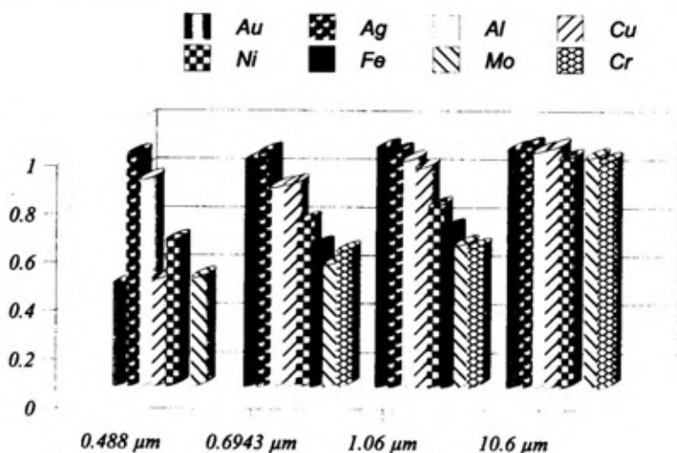
Sl. 7 – Reflektivnost nekih metala za različite talasne dužine laserskog zračenja
