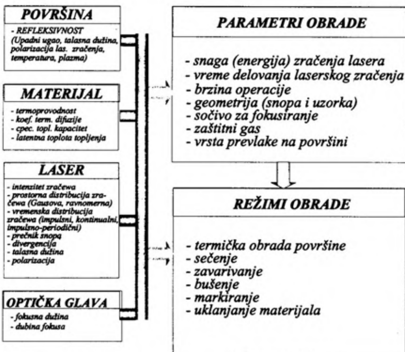
Sl. 8 – Faktori koji definišu režime obrade materijala
