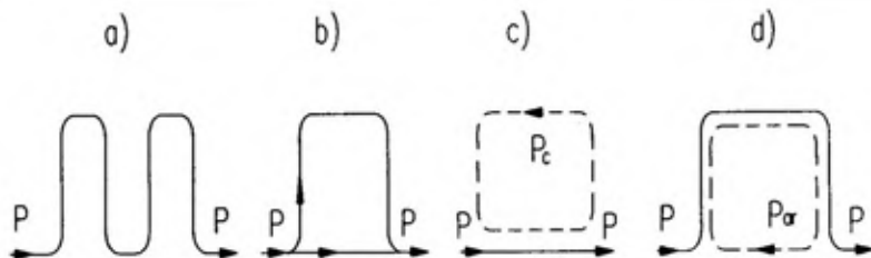
Sl. 4 – Mogući tokovi snage u planetarnom prenosniku
