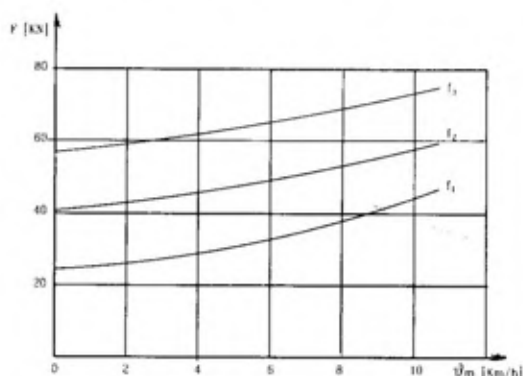
Sl. 7 - Zavisnost vučne sile od relativne brzine tenka
