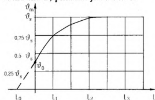
Sl. 2 – Promena relativne brzine kretanja tenka
