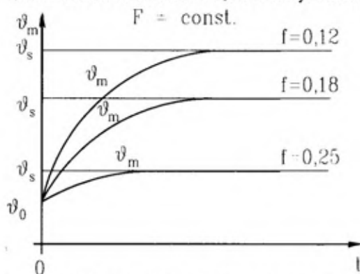
Sl. 3 – Uticaj koeficijenta otpora kotrljanja na ubrzanje tenka
