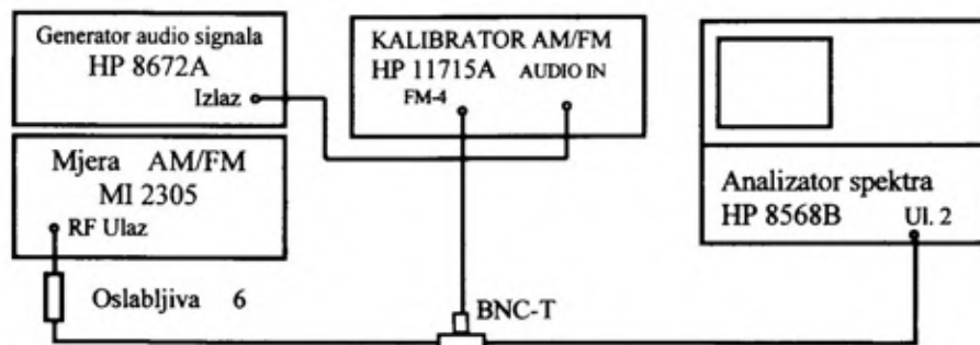
Sl. 4 – Blok-šema povezivanja mjernih uređaja za provjeru devijacije FM
