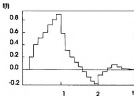
Sl. 7 – Primer postepenog aproksimiranja funkcije
