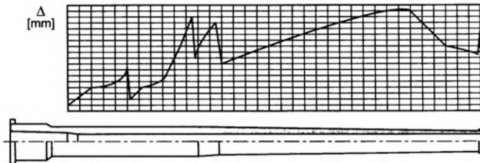
Sl. 4 – Načelni izgled dijagrama graničnih mehaničkih oštećenja spoljašnje površine cevi (bez prslina)
