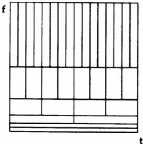
Sl. 6 – Primer baze talasne transformacije u vremensko-frekvencijskoj ravni
