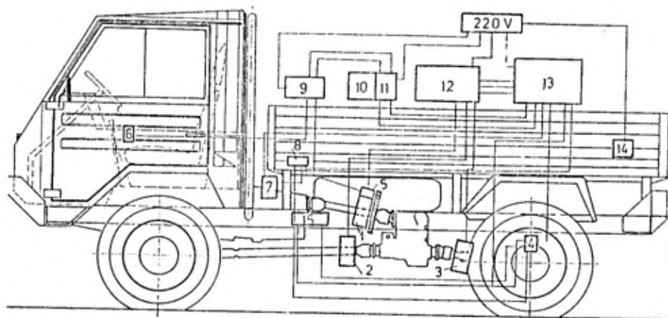
Sl. 5 — Blok-šema mernog sistema:
