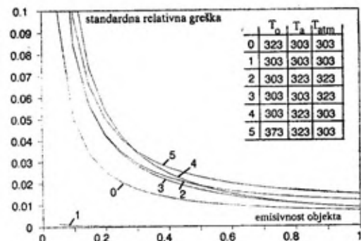
Sl. 5 — Zavisnost relativne standardne greške od emisivnosti objekta za različite vrednosti T_o , T_a , T_{atm}
