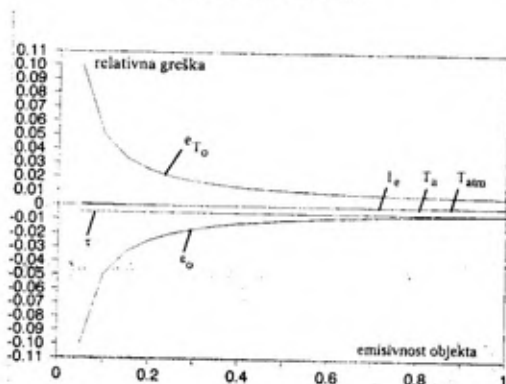
Sl. 4 — Zavisnost relativne greške od emisivnosti objekta
