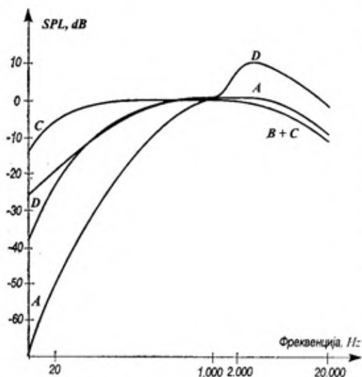
Sl. 1 — Korekcione karakteristike A, B, C
