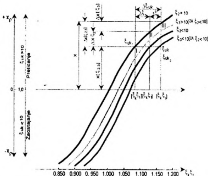
Sl. 4 — Zavisnost sile pogona i koeficijenata preticanja i zaostajanja pogonskih točkova pri kretanju u krivini po neravnoj podlozi
