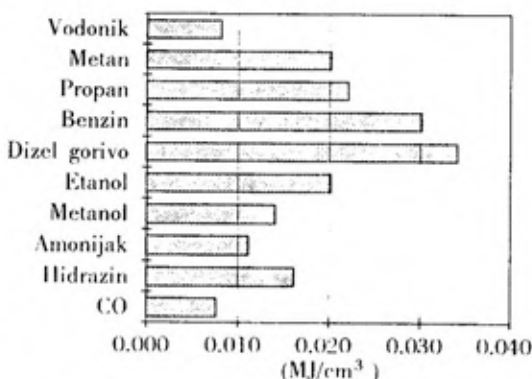
Sl. 2 — Toplotna gustina goriva po jedinici zapremine
