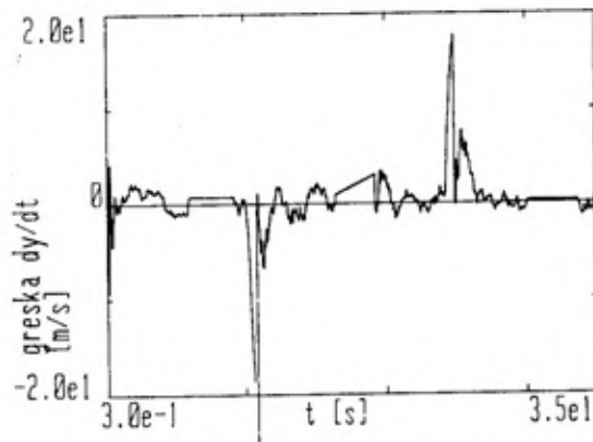
Sl. 8 — Greška ocene y-komponente brzine
