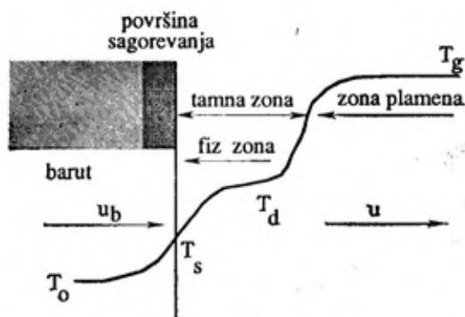
Sl. 2 — Pojednostavljen model sagorevanja baruta
