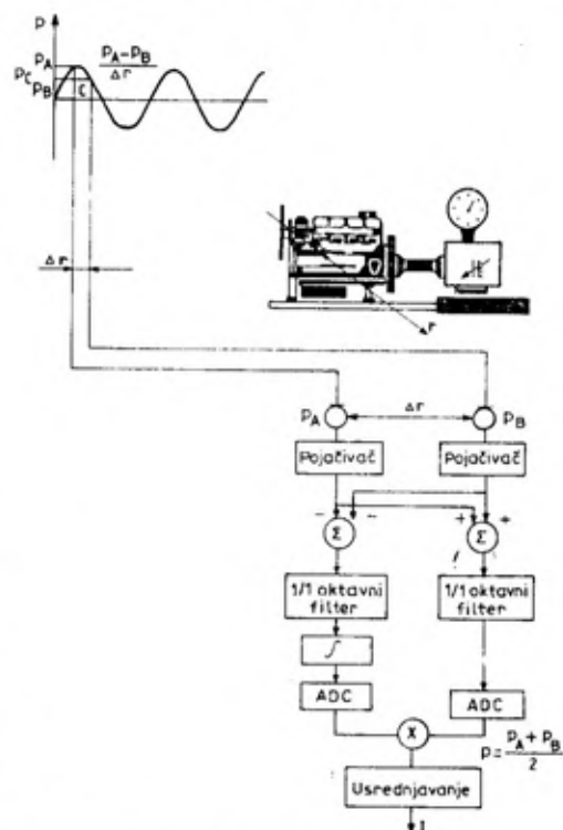
Sli. 6 — Šema toka mernog signala zvučnog intenziteta
