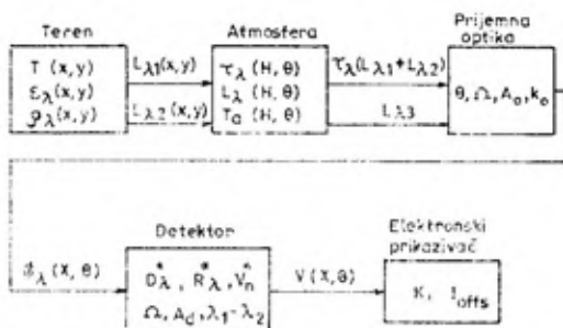
Sl. 1 — Uprošćeni model za formiranje slike terena
