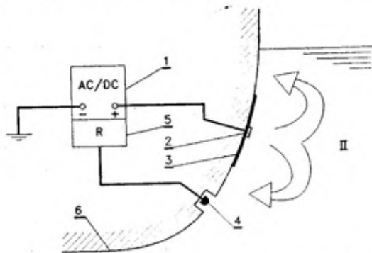
Sl. 2 — Principijelna šema uređaja AKZ 1 — stanica AKZ, 2 — anoda, 3 — okolaoanodni ekran, 4 — referentna elektroda, 5 — regulaciona jedinica, 6 — trup broda
