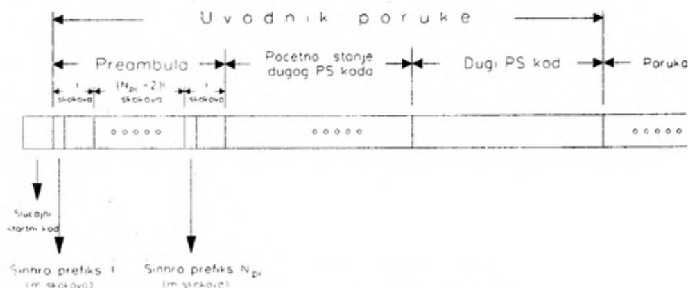
Slika 1 — Struktura uvodnika poruke
