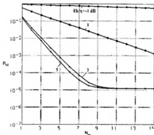
Sl. 7 — Minimum verovatnoće nedetekcije u funkciji broja pasivnih korelatora, odnos E_b/\eta je parametar ( P_M \leq 10^{-8} ; F = 0,15 ; df = 25 dB; D = 64 ; m = 16 ; L = 320 ; N_2 = 11 ; k = 512 ; N_{ac} = 1 )
