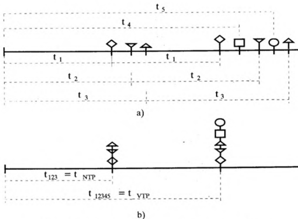
Sl. 3 — Objedinjavanje pojedinih operacija u tehničke preglede t_1, t_2, \dots, t_i — periodičnost izvođenja pojedinih operacija t_m, \dots, i — periodičnost izvođenja objedinjenih i -operacija t_{NTP}, t_{VTP} — periodičnost nižeg i višeg pregleda
