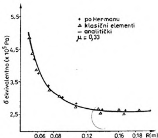
Sl. 13 — Zavisnost ekvivalentnog napona od spoljašnjeg poluprečnika
