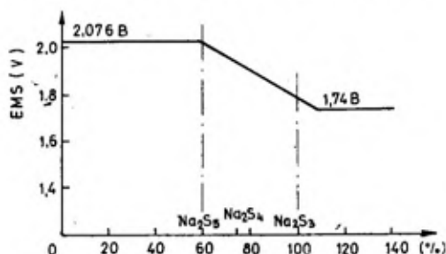
Sl. 6 — Pražnjenje u odnosu na \text{Na}_2\text{S}
