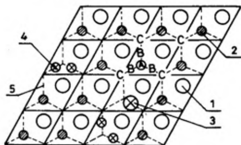
Sl. 5 — Struktura provodne površine \beta -glinica-keramik
