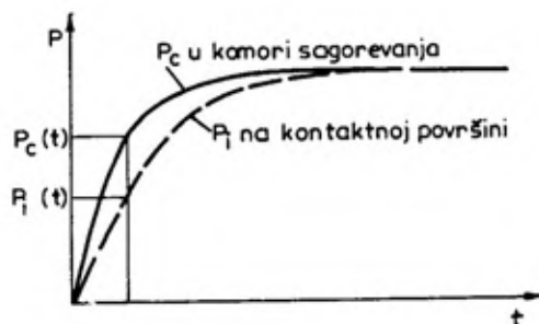
Sl. 2 — Porast pritiska u fazi pripaljivanja
