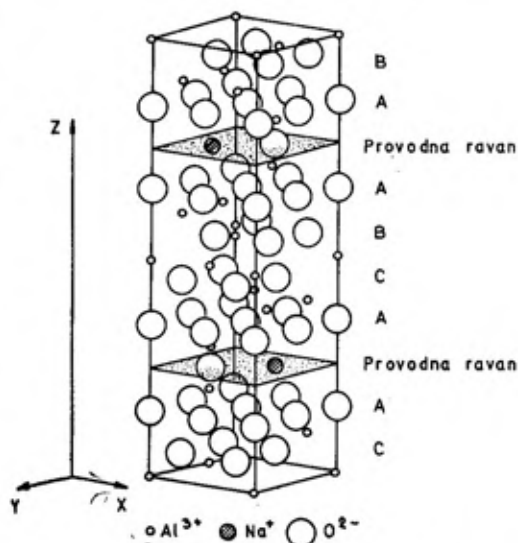
Sl. 4 — Idealizovana elementarna ćelija \beta -glinice
