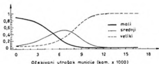
Sli. 5 — Verovatnoća utroška municije po klasama za divizion 122 mm
