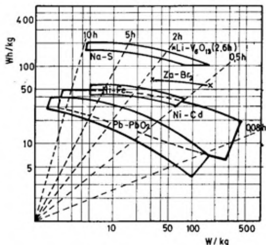
Sl. 1 — Ragone-dijagram
