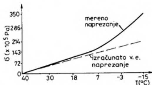
Sl. 9 — Promena napona sa temperaturom
