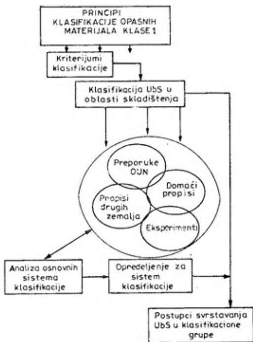
Sl. 2 — Principi klasifikacije opasnih materija
