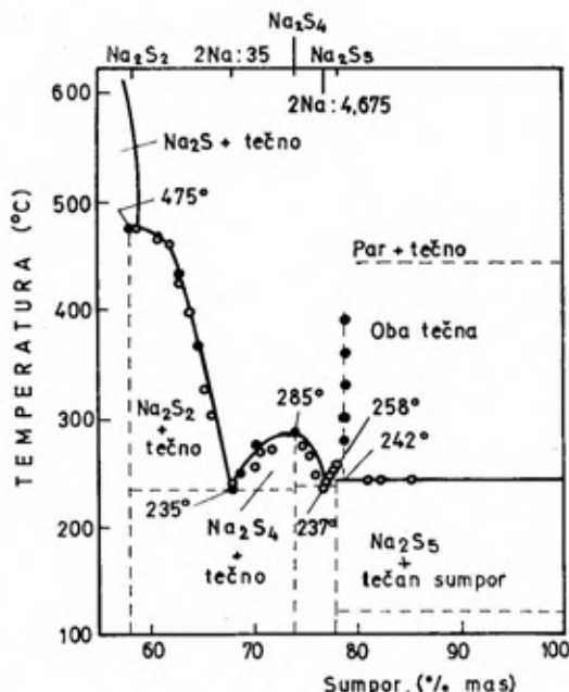
Sl. 3 — Dijagram stanja \text{Na}_2\text{S}-\text{S}
