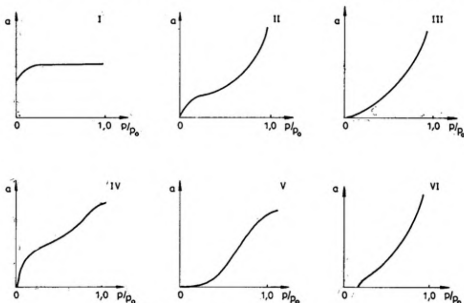
Sl. 2 — Tipovi adsorpcionih izoterma
