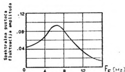
Sl. 5 — Zavisnost spektra fluktuacija amplituda reflektovanih signala od aviona u letu
