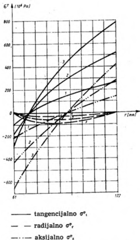
Sl. 4 — Naprezanje usled temperature
