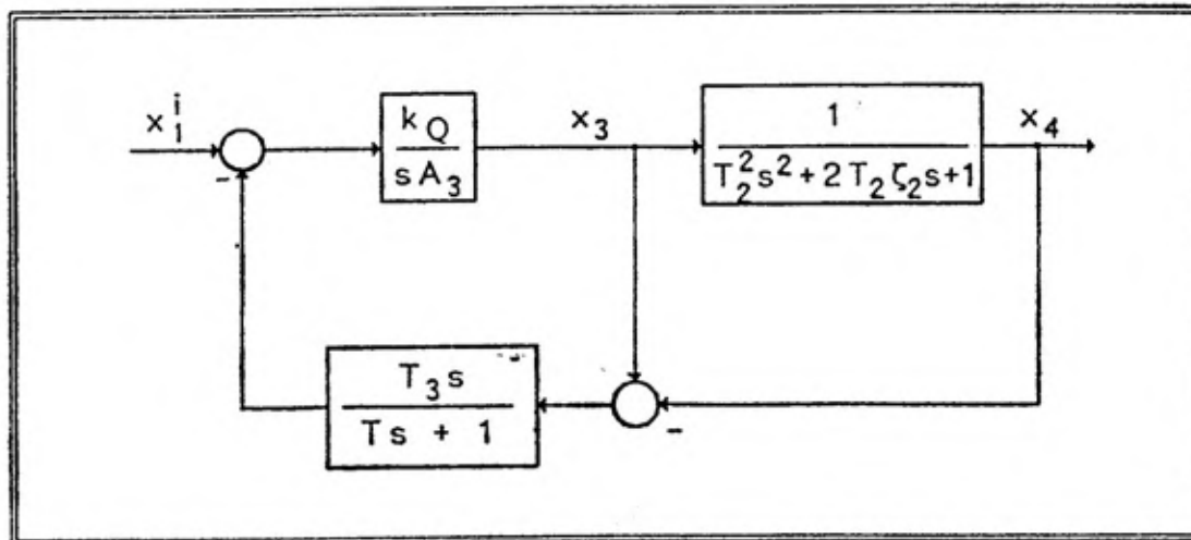
Sl. 4 — Transformirana strukturna shema
