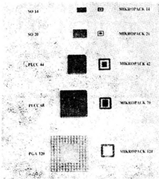
„Bild 1: Vergleichender Anschauungsbild haben ICs in der MIKROPACK-Bauform deutlich vorteilhaft.“
