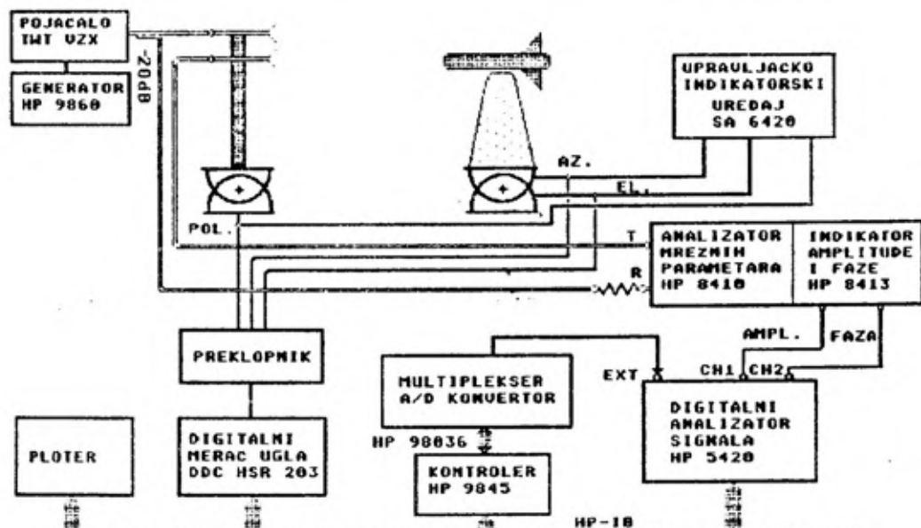
Sl. 2 — Merni sistem za merenje i analizu »bleštavih tačaka« rotirajućeg cilja
