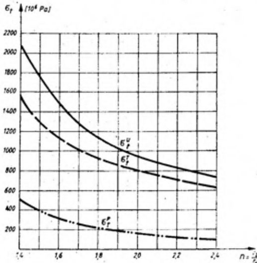
Sl. 1 — Tangencijalno naprezanje na radiju- su r_1
