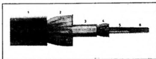
Sl. 8 — Optički širokopojasni laki kabl sa dva vlakna za vojne namene (prema standardu američke armije), male mase i faktora prigušenja (slabljenja) sa visokom termičkom tolerancijom (od -55^{\circ} do +85^{\circ}\text{C} ):
