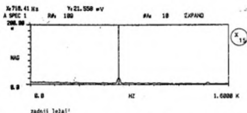
D.3. Dijagram spektra vibracija reklamiranog motora ASTAZOU XIV M na jednom režimu iz Programa ispitivanja nakon otklanjanja uzroka vibracija
