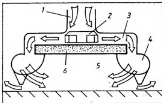
Sl. 4 — Sema rasporeda amfibijskog čamca na vazdušnom jastuku sa dvoslojnom gipkom ogradom:
