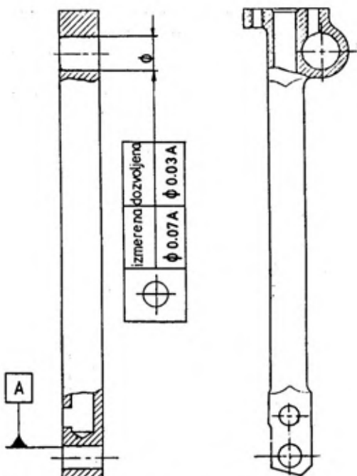
Sl. 5 — Izmerena odstupanja na pačku zadnjeg ležaja GTM ASTAZOU XIVM
