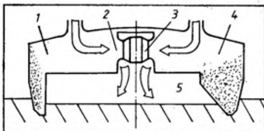
Sl. 5 — Sema opšteg skegovog čamca na vazdušnom jastuku:
