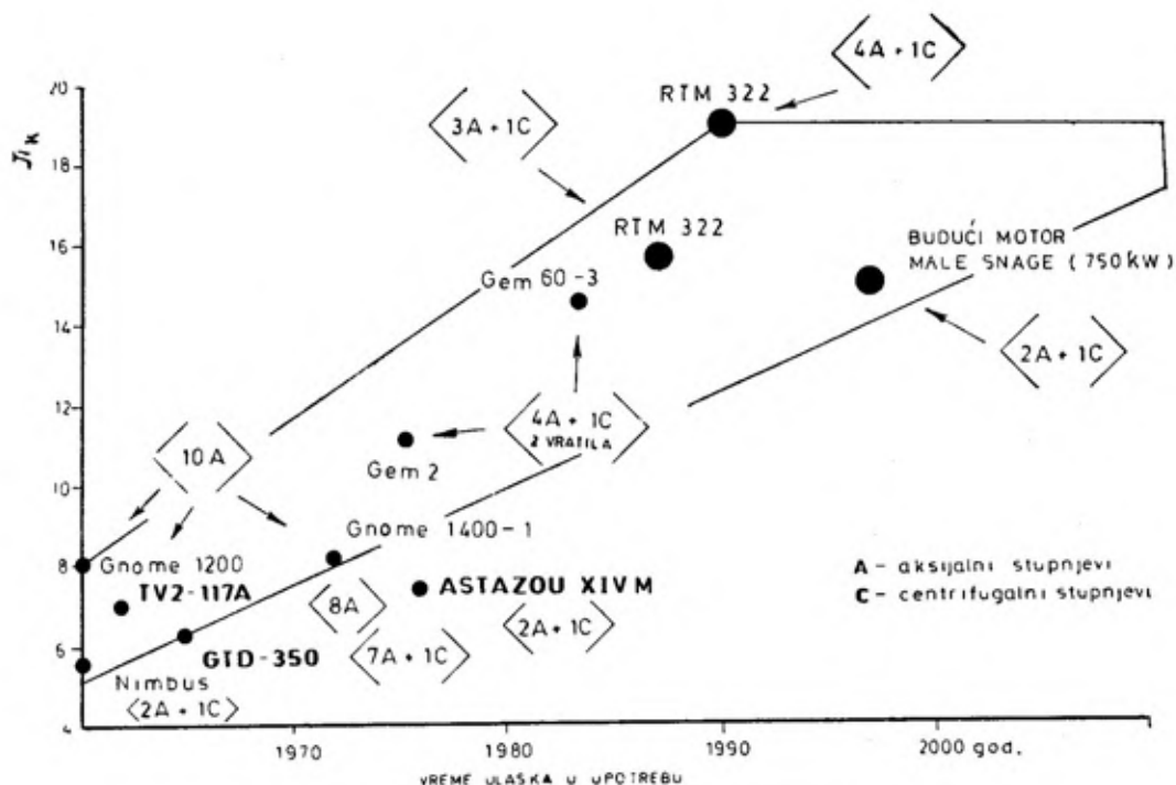
Sl. 3 — Trend rasta stepena sabijanja kompresora ( \pi_k ) GTR
