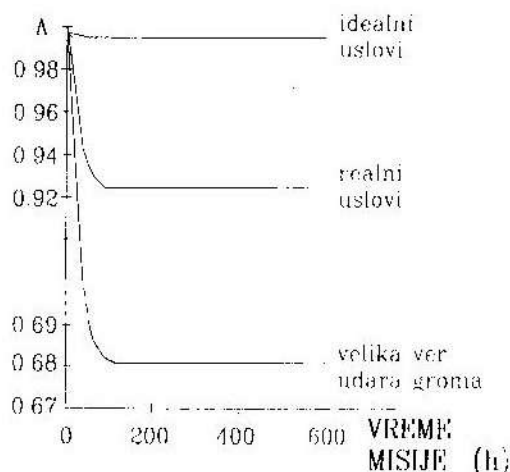
Sl. 7 — Raspoloživost integrisanog elektronskog sistema sa tri redundantne magistrale u uslovima bez smetnji, u realnim radnim uslovima i u uslovima velike verovatnoće udara groma
