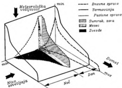
Sl. 1 Međusobni odnos mogućnosti dnevnih (optičkih) sprava, pasivnih sprava i termovizijskih uređaja
