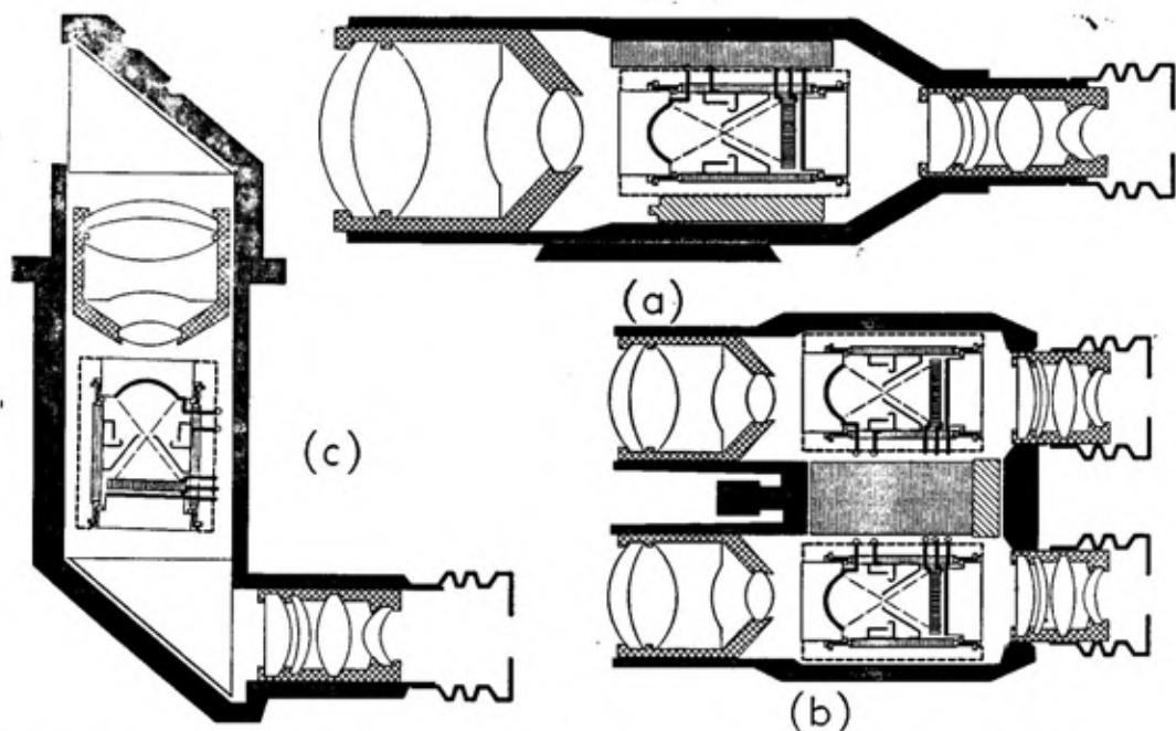
Sl. 14 Primeri najčešćih primena pojačavača slike u vojnim optoelektronskim spravama
