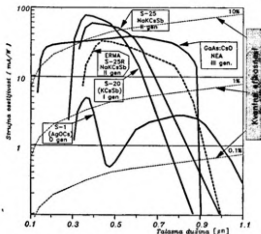
Sl. 8 Spektralne zavisnosti strujne osetljivosti najčešće korišćenih tipova fotokatoda u pojačivačima slike
