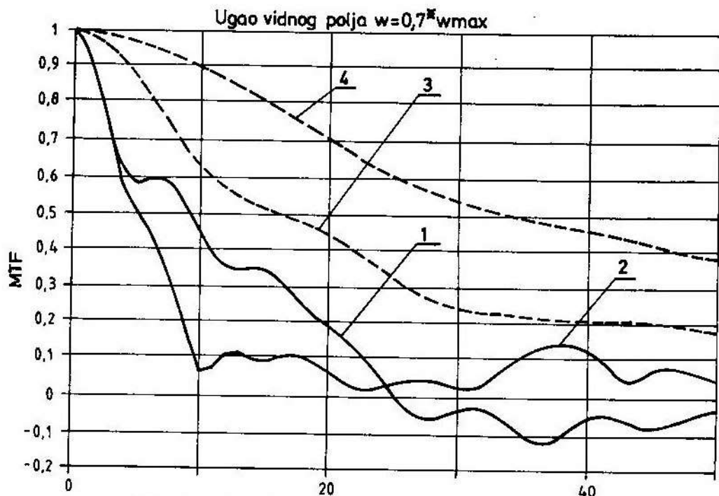
Sl. 2b Uporedni prikaz MTF-a za polazni i optimizirani optički sistem (za 0,7 od ugla vidnog polja)
