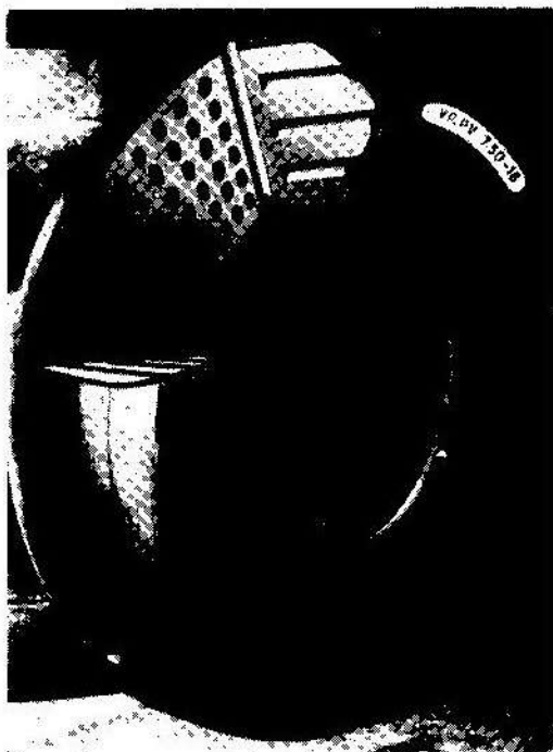
Sl. 4 Delimični presek neranjive gume sa ćelijastim umetkom HUTCHINSON VP-PV.
