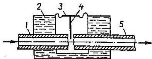
Sl. 1 Zaslonski davač pritiska:
