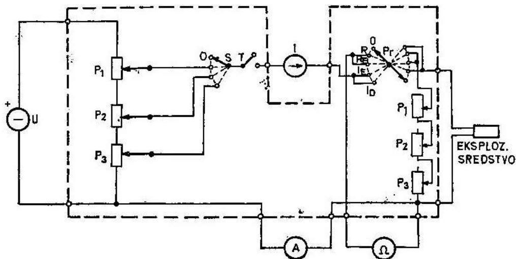
SL. 3 Metoda sa struinim generatorom
