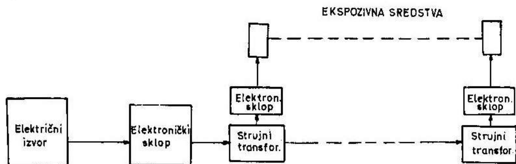
Sli. 4 Blok shema metode sa induktivnim strujnim transformatorima
