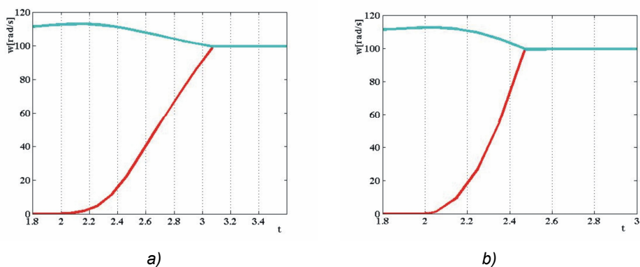
Slika 12 – Rezultati simulacije za a) N_r = 4 i b) N_r = 12
