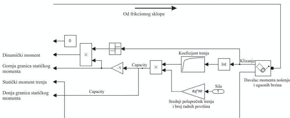
Slika 8 – Model trenja
