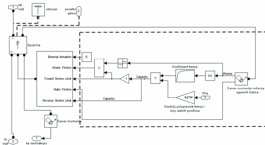
Slika 5 – Model za simulaciju rada višelamelastih frikcionih sklopova
